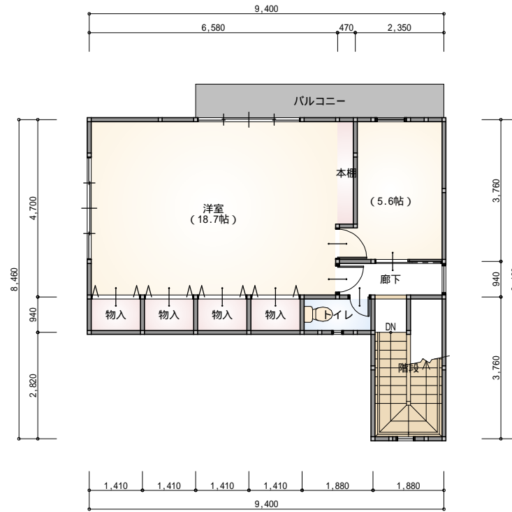
2階 平面図 S : 1 / 140
